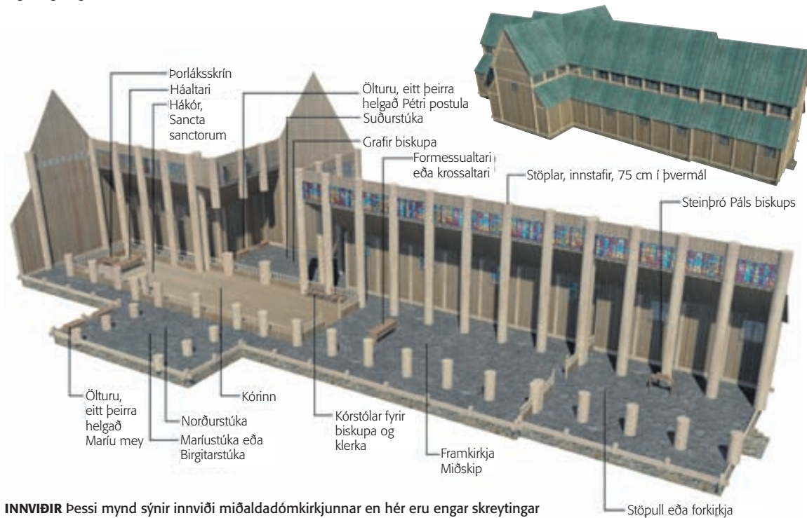
MIÐALDADÓMKIRKJA Í SKÁLHOLTI Tölvugerð mynd sem sýnir kirkjuna með koparþaki að mestu og tiltölulega stórum gluggum með steindu gleri. Ákvarðanir um endanlegt útlit kirkjunnar hafa ekki verið teknar. Myndirnar hér fyrir neðan sýna ýmsar útgáfur af hugsanlegu útliti kirkjunnar. Dómkirkjurnar íslensku voru einstæðar í evrópski byggingarsögu og voru um tíma stærstu timburhús á Norðurlöndum.
