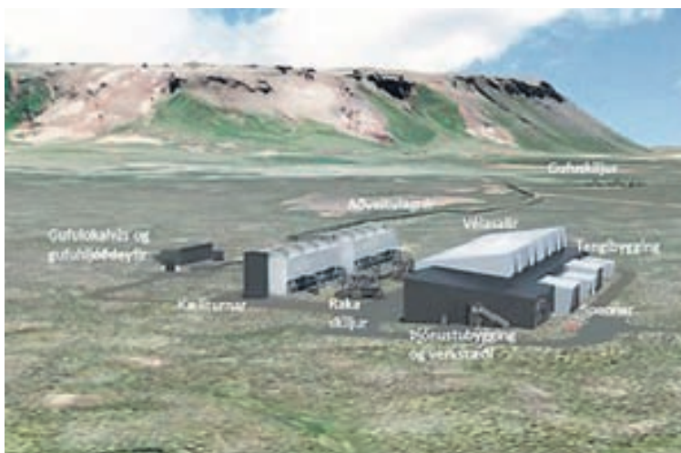
PEISTAREYKJIR Húsin rúma tvær 45 MW aflvélar – óvíst er hvenær ráðist verður í uppsetningu seinni vélarinnar. MYND/LANDSVIRKJUN
